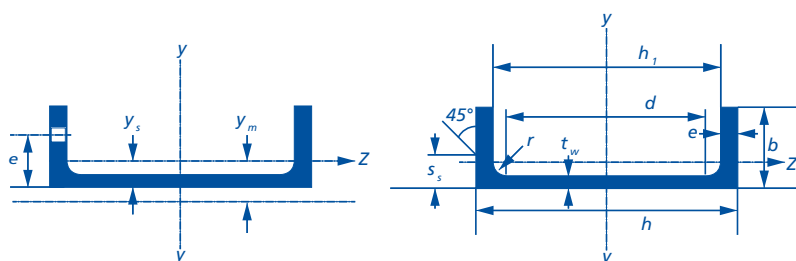
UPE SELON NF EN 10279
